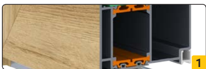
TROJKOMOROVÉ PROFILY S HĽBKOU 77 MM S TEPELNOIZOLAČNÝMI PRESTÁVKAMI
