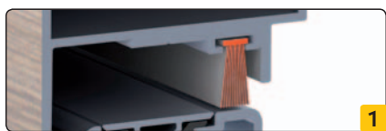
PRÍDAVNÉ ŠTETINOVÉ TESNENIE TESNÍ MEDZERU MEDZI KRÍDLOM A PRAHOM
